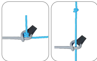
Gráfico 2. Conexión del acelerador mediante lazada tipo “Kite” (sin gancho Brummel). El suspenso azul es de la silla y el gris, de la banda.
