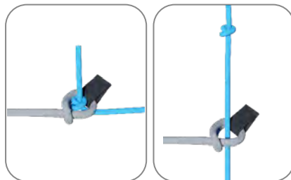
Gráfico 2. Conexión del acelerador mediante lazada tipo “Kite” (sin gancho Brummel). El suspente azul es de la silla y el gris, de la banda.
