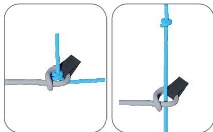
Diagramme 2. Connexion de l'accélérateur avec tête d'alouette (sans crochets Brummel). La ligne bleue est celle de la sellette, et la grise, de l'élévateur.
