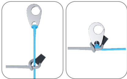
Gráfico 1. Conexión del acelerador mediante el paso del gancho Brummel. El suspente azul es de la silla y el gris, de la banda.
